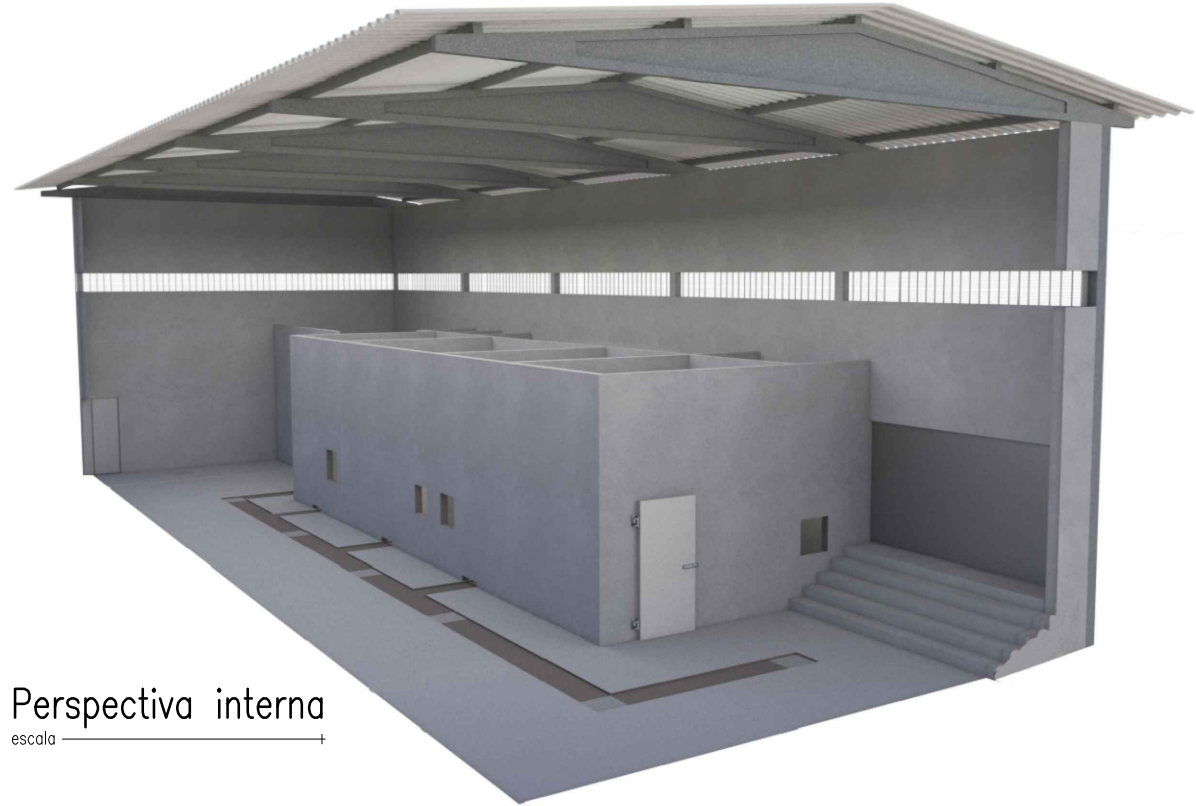
Perspectiva interna escala 1/75
