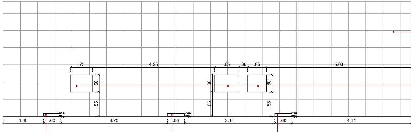
Vista 01 – Aberturas escala 1/75
