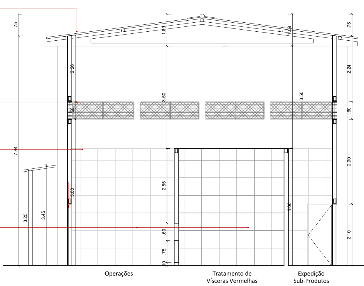
Corte BB – Galpão escala 1/75
