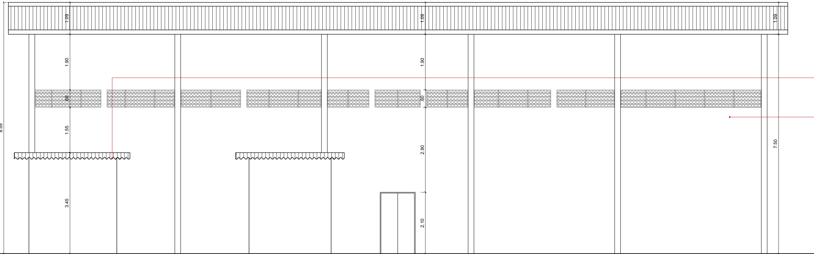
Fachada Lateral Esquerda – Galpão escala 1/75
