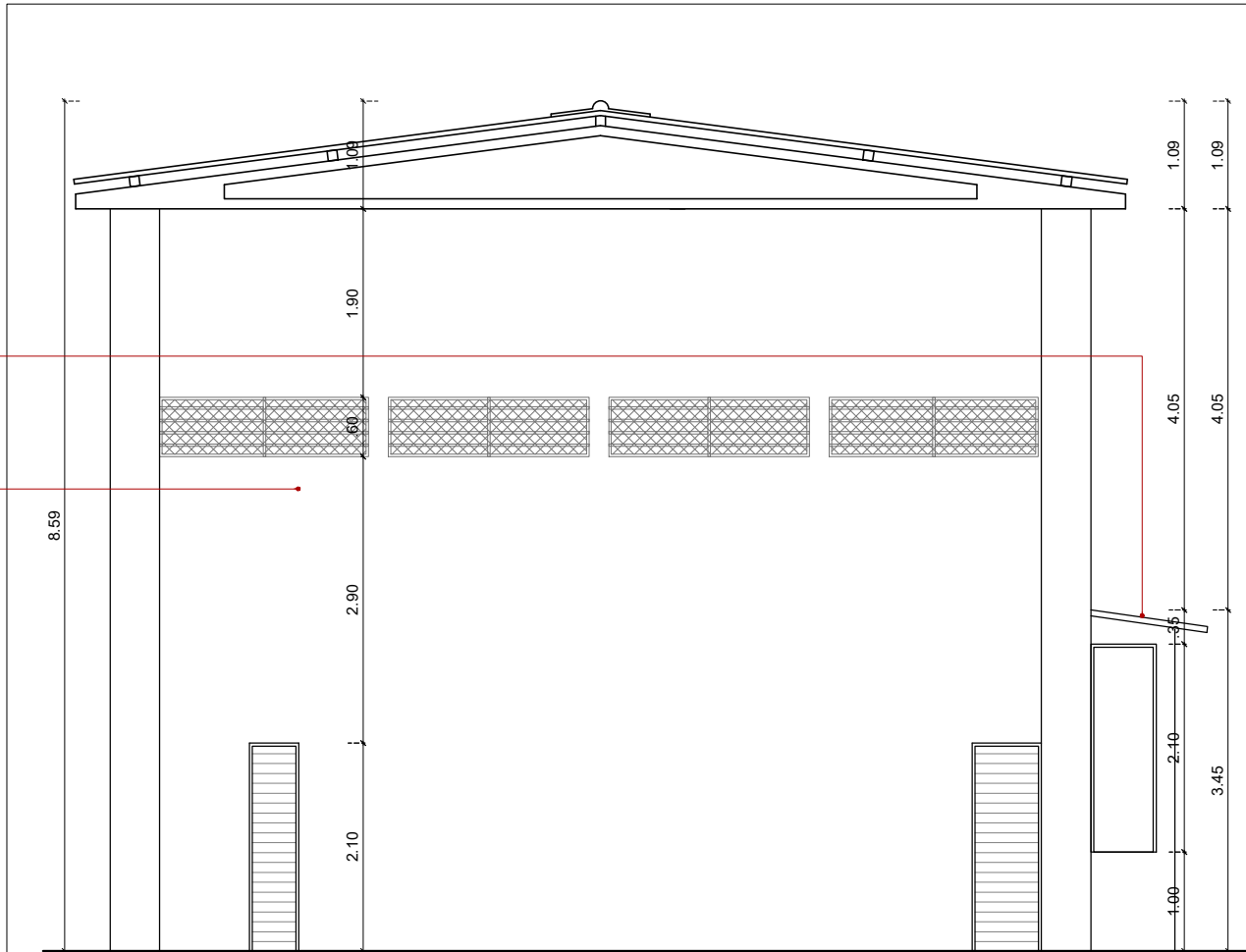
Fachada Frontal – Galpão escala 1/75
